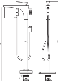
N3645YL 落地式浴缸龙头 黄铜 枪灰 暗装预埋盒
