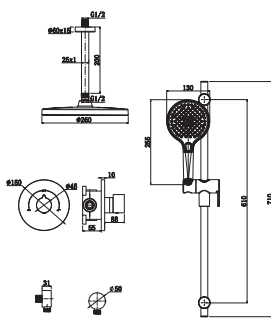
L6511YF 入墙式两功能淋浴套装 黄铜 镀铬
