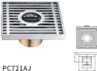
PC721AJ 地漏 100*100mm 黄铜+深水封 镀铬
