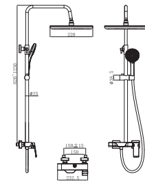
L3601ZS 三功能淋浴套装 黄铜 镀铬
