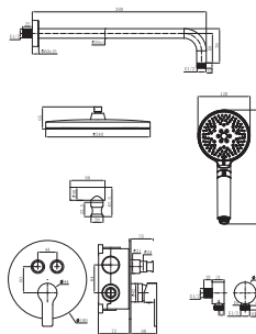
L6261YF 入墙式两功能淋浴套装 黄铜 镀铬
