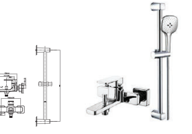
L2631GE 两功能淋浴套装 黄铜 镀铬
