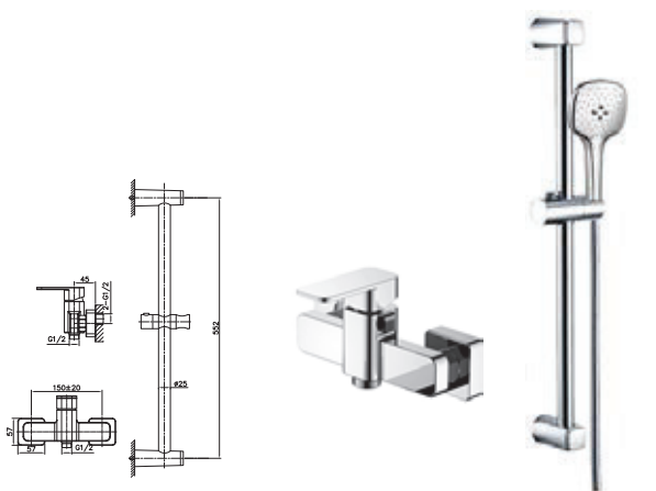
L1691GE 单功能淋浴套装 黄铜 镀铬
