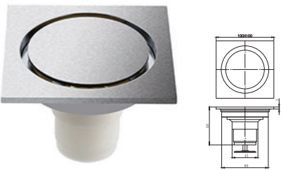
PC543AJ 地漏 100*100mm 黄铜 镀铬
