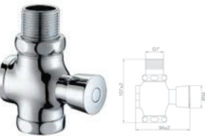
PC211CW 按式小便冲洗阀 黄铜 镀铬
