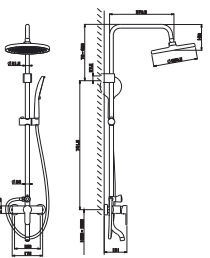
L3162PD 三功能淋浴套装 黄铜 哑黑
