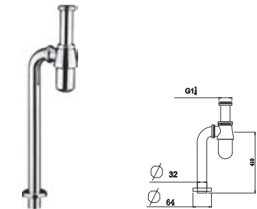
PS671MK 地排排水管 304不锈钢 镀铬
