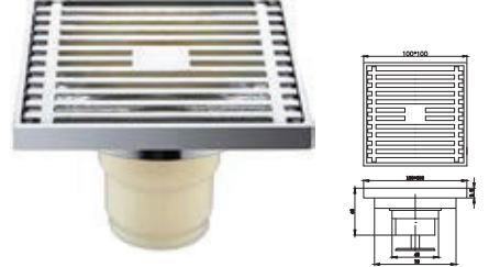
PC611AJ 地漏 100*100mm 黄铜+深水封 镀铬
