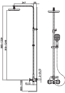
L2621GE 两功能淋浴套装 黄铜 镀铬
