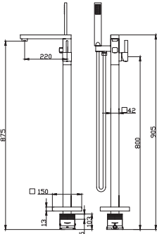
N3511YL 落地式浴缸龙头 黄铜 镀铬 暗装预埋盒
