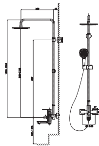
L3691GE 三功能淋浴套装 黄铜 镀铬
