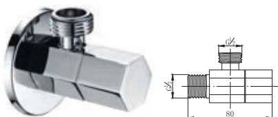
PC411AJ 角阀 黄铜 镀铬
