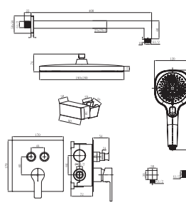
L6271YF 入墙式两功能淋浴套装 黄铜 镀铬
