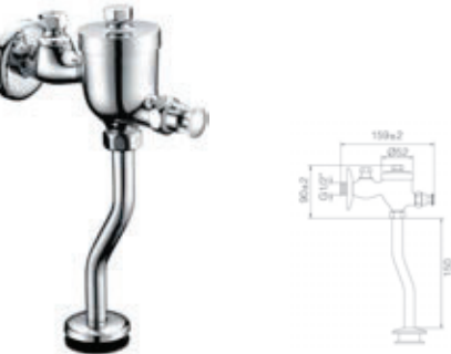
PC221CW 按式小便冲洗阀 黄铜 镀铬
