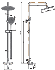
L2731WB 两功能淋浴套装 黄铜 镀铬
