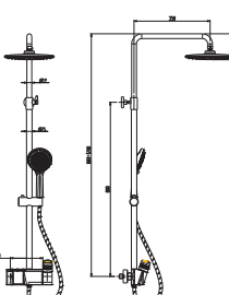
L3035YF 三功能淋浴套装 黄铜 枪灰
