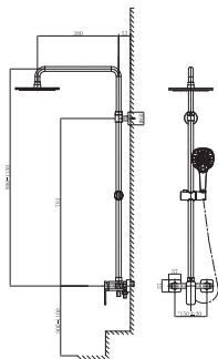
L2691GE 两功能淋浴套装 黄铜 镀铬
