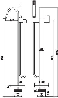
N3621YL 落地式浴缸龙头 黄铜 镀铬 暗装预埋盒
