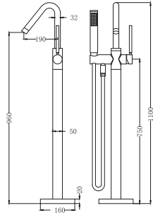
N3852YL 落地式浴缸龙头 黄铜 哑黑 暗装预埋盒
