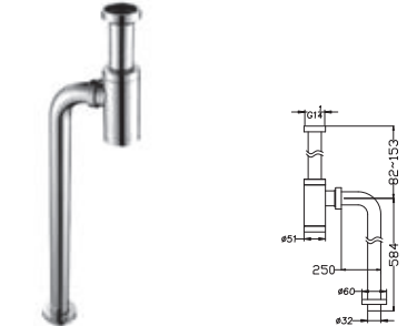
PC211MK 地排排水管 黄铜 镀铬
